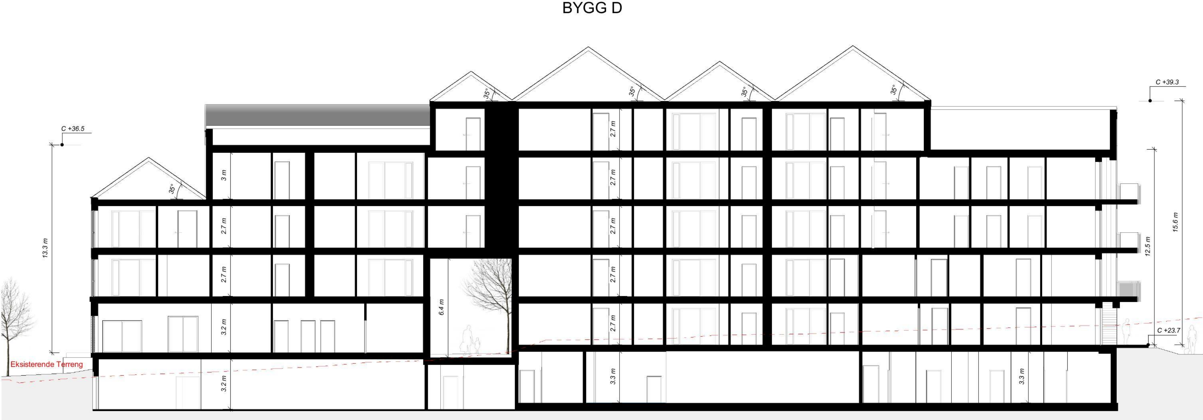
Lengdesnitt bygg D 1 : 200
